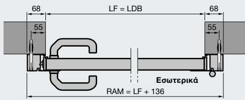
Πλαϊνή πόρτα με απλή κάσα αλουμινίου τύπος προφίλ 1 Τοποθέτηση πίσω από το άνοιγμα
