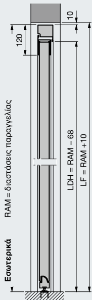
Πλαϊνή πόρτα με απλή κάσα αλουμινίου προφίλ τύπου 2 Τοποθέτηση ανάμεσα στο άνοιγμα
