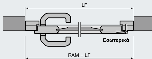
Πλαϊνή πόρτα από μασίφ ξύλο Τοποθέτηση ανάμεσα στο άνοιγμα
