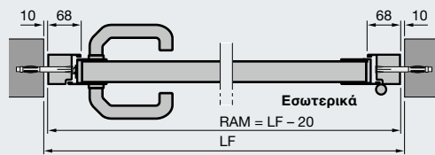
Πλαϊνή πόρτα με απλή κάσα αλουμινίου προφίλ τύπου 2 Τοποθέτηση ανάμεσα στο άνοιγμα
