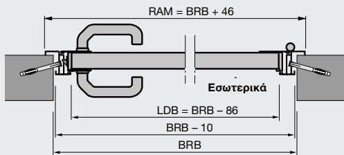
Πλαϊνή πόρτα με γωνιακή κάσα αλουμινίου προφίλ τύπου 3 Άνοιγμα προς τα έξω
