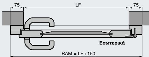
Πλαϊνή πόρτα από μασίφ ξύλο Τοποθέτηση πίσω από το άνοιγμα
