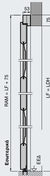
Πλαϊνή πόρτα από μασίφ ξύλο Τοποθέτηση πίσω από το άνοιγμα
