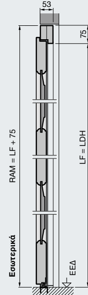
Πλαϊνή πόρτα από μασίφ ξύλο Τοποθέτηση ανάμεσα στο άνοιγμα
