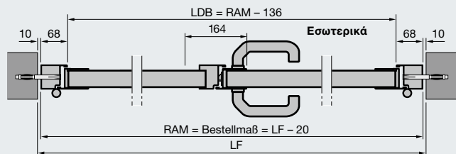
Δίφυλλη πλαϊνή πόρτα με απλή κάσα αλουμινίου προφίλ τύπου 2 Τοποθέτηση ανάμεσα στο άνοιγμα
